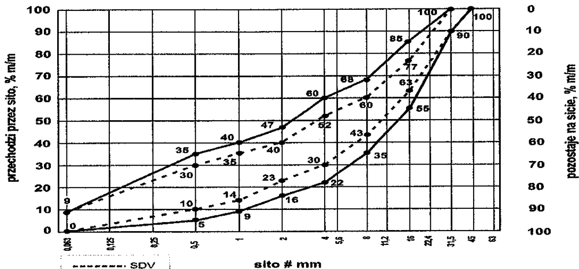
Rysunek 3. Mieszanka niezwiązana 0/31,5 do warstwy podbudowy zasadniczej
