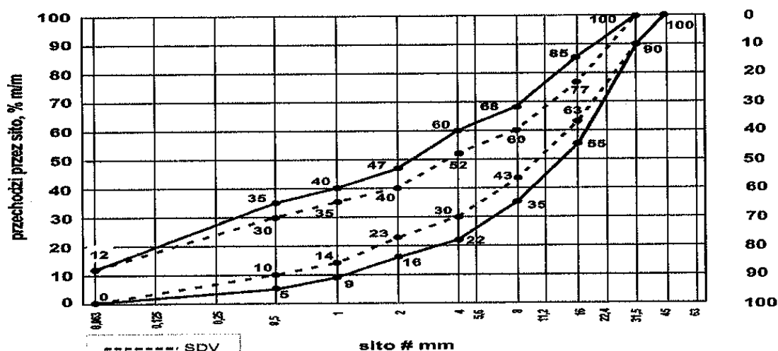
Rysunek 2. Mieszanka niezwiązana 0/31,5 do warstw podbudowy pomocniczej
